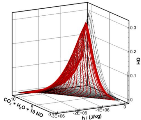
Abb. 1: REDIM (schwarzes Gitter) sowie Profile (rot) einer Verlöschung an einer Wand
